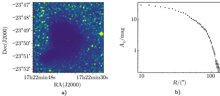
注: a) 数字巡天 (Digitized Sky Survey) 的光学图像,红色的“+”号表示尘埃消光最大的位置; b) 尘埃消光的径向分布 [4] 。
