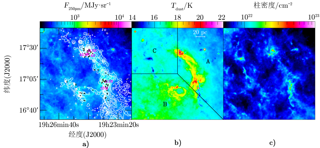
注: a) 背景为 250\ \mu\text{m} 尘埃发射, 等值线为 CO 强度积分图。等值线始于 3\sigma ( 1\sigma=0.3\ \text{K}\cdot\text{km}\cdot\text{s}^{-1} ), 步长为 3\sigma , 椭圆为致密团块。4 个大质量团块 (15, 26, 42, 43) 以及与 II 型甲醇脉泽成协 (15, 43, 52) 的团块用方框标出。b) 温度分布图中的 3 个区域用 A, B, C 标出, 用于分析尘泡的径向流量分布。
