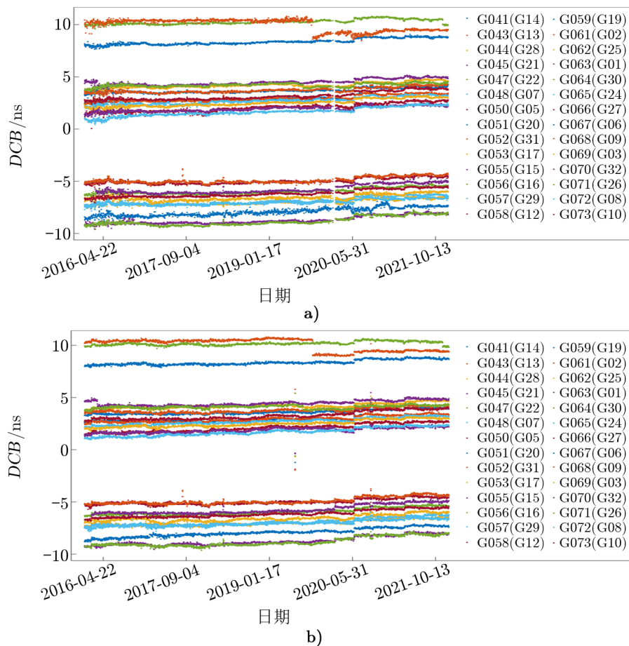
图 5 GPS 卫星未统一基准的 C1C-C2W 频间偏差时间序列图
