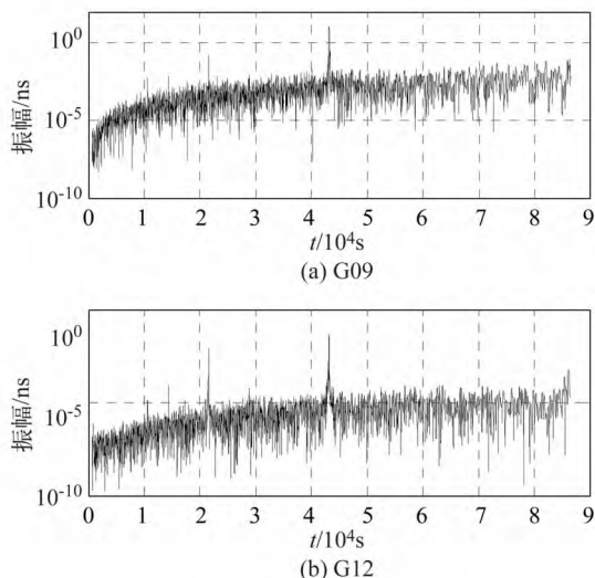
图3 GPS 9号、12号卫星钟差频谱图
